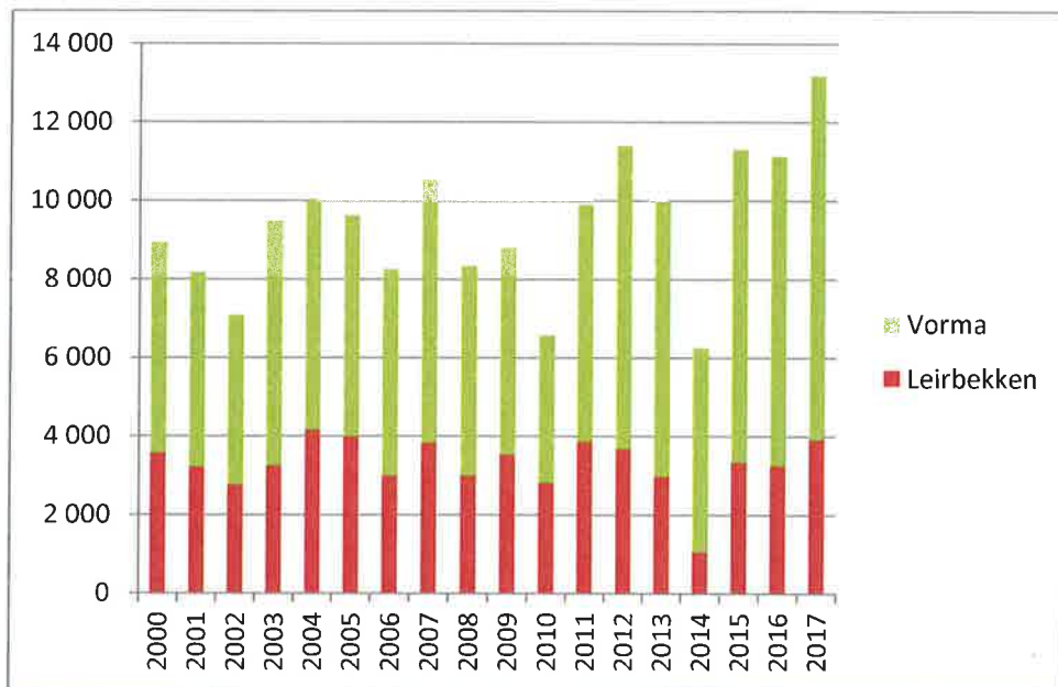
Figuren viser årlig kraftproduksjon i perioden 2000-2017
