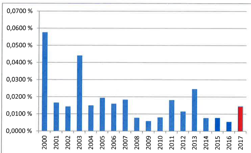
Figuren viser utviklingen i driftssikkerhet (målt i andel ikke levert energi av totalt overført energi forårsaket av avbrudd i Orkdal Energis strømnnett) i perioden 2000-2017.
